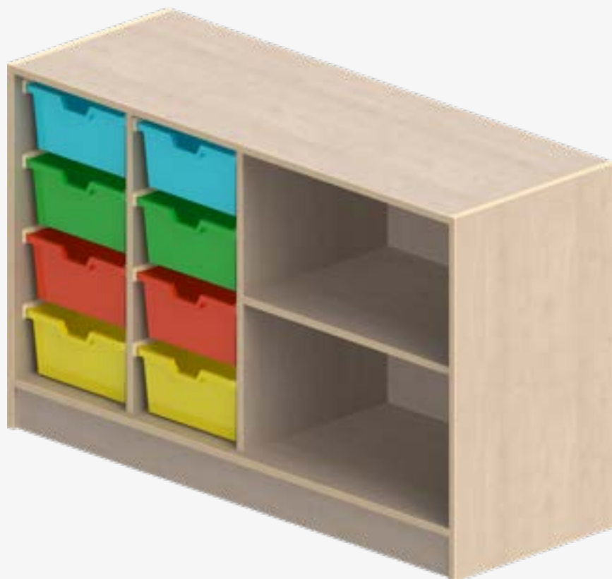
MOB4/8L dělená, otevřený regál levá 8× box F2 1387 × 850 × 500 mm
